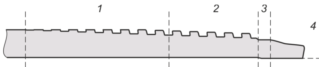
а) – Поверхность резьбового соединения ниппеля
