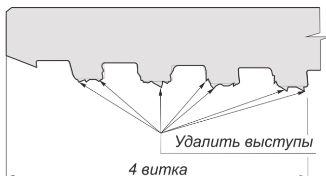
б) – Поверхность резьбового соединения муфты
